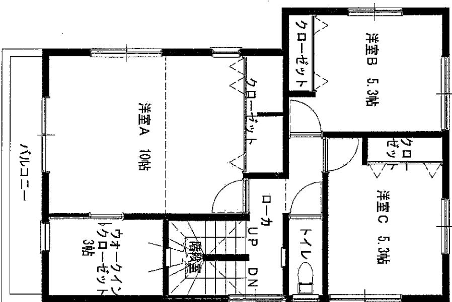
2階平面図
